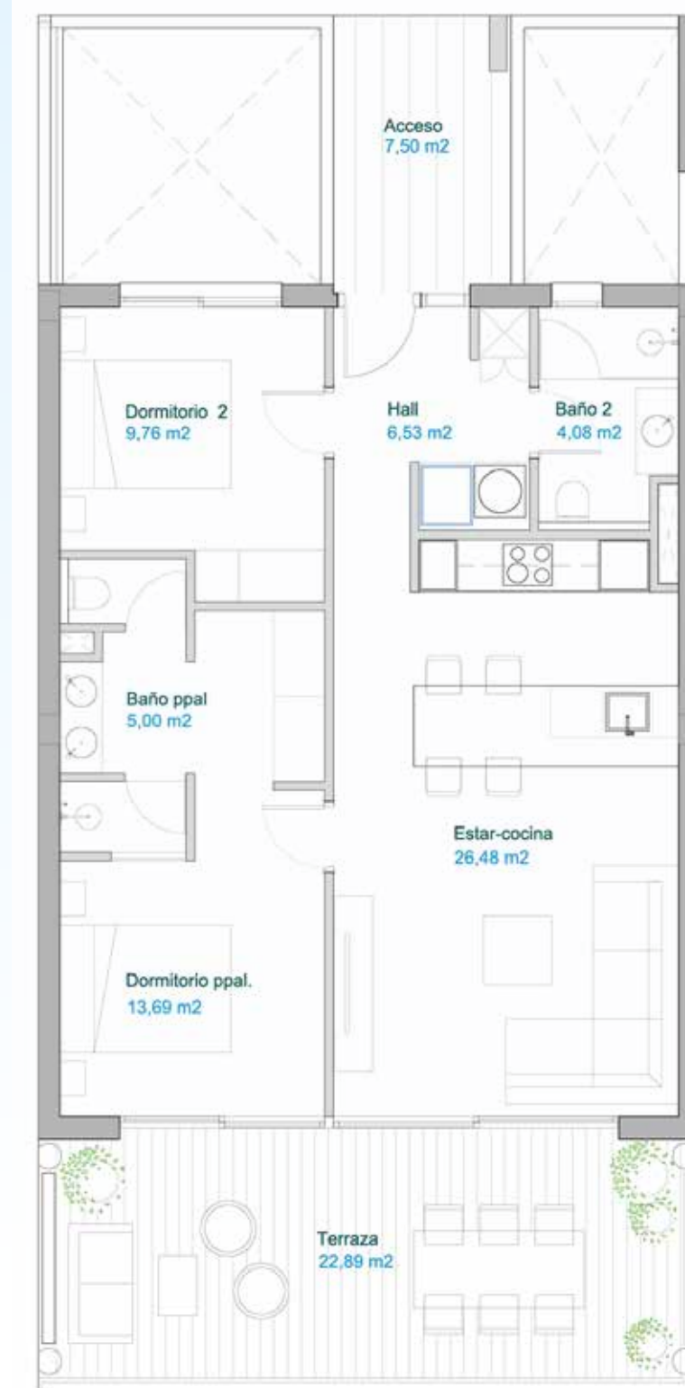
PLANTA. Escala_1/80
